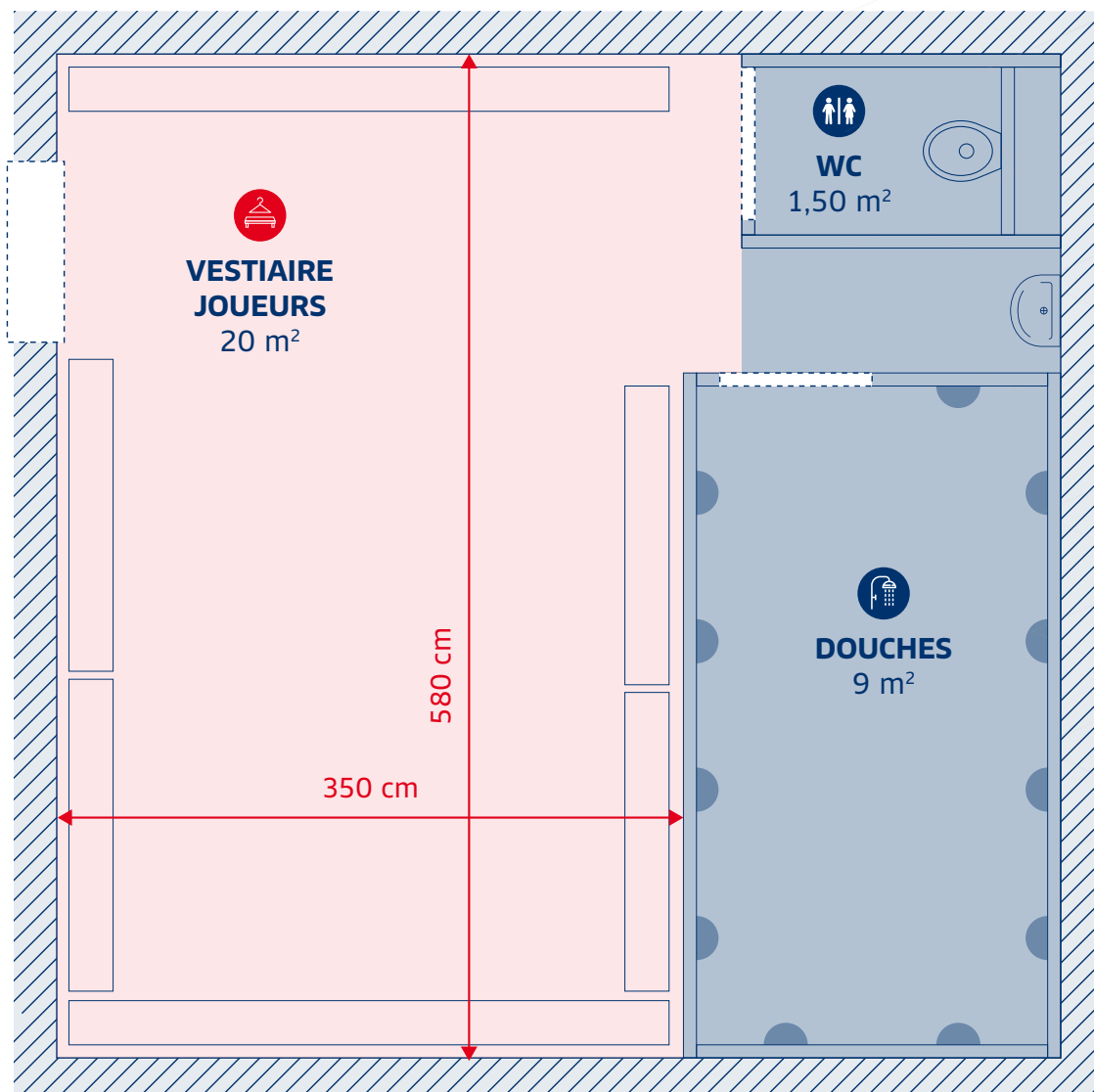
► Schéma n°27 : exemple de plan de vestiaire
