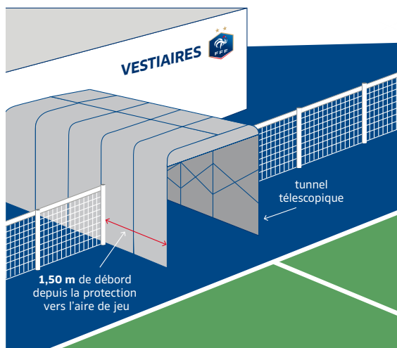
▶ Schémas n°32 : exemples de dispositifs de protection entre les vestiaires et le terrain
