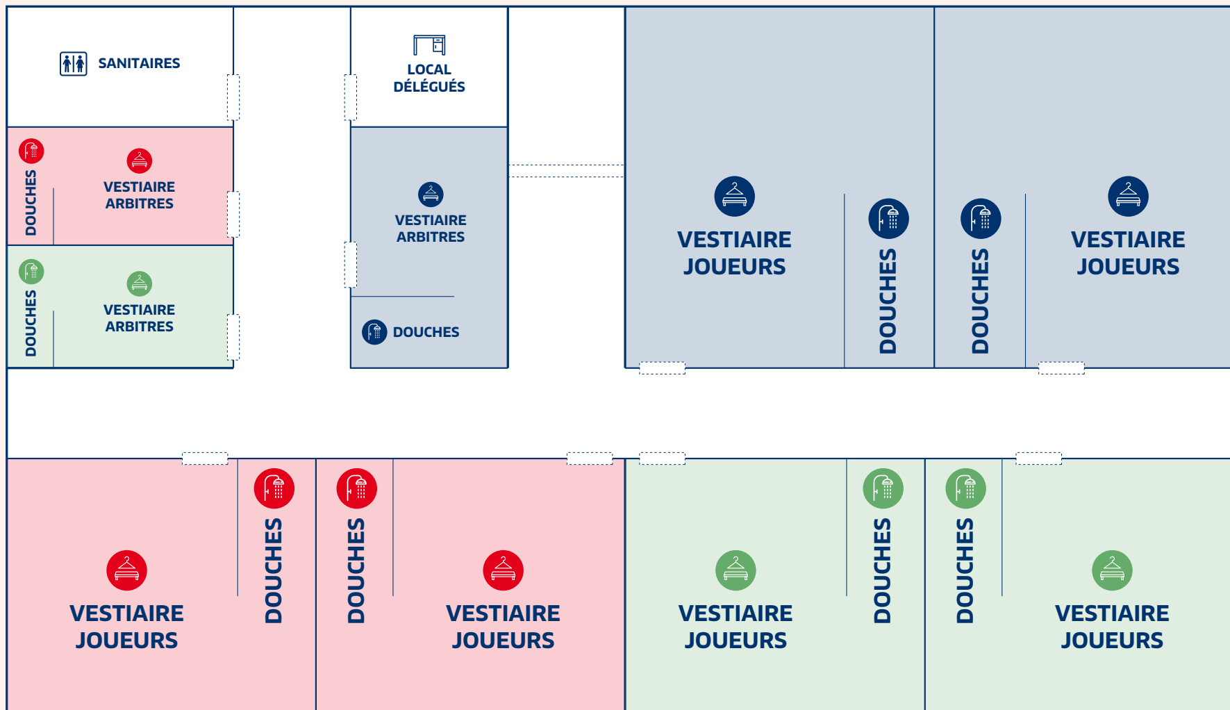
🔗 Schéma n°26 : principe d'affectation de locaux à un terrain pour former une installation
