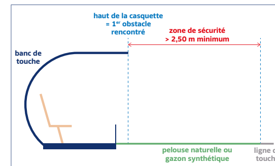
Vue latérale
