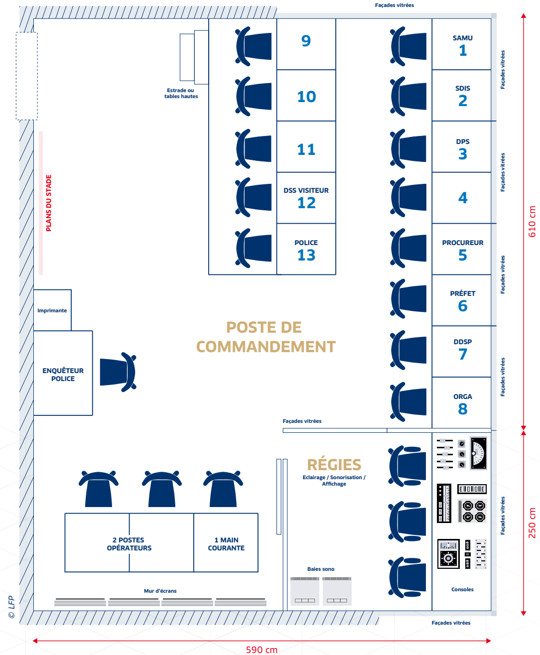
► Schéma n°36 : principe d'organisation du volume d'un PCM (dimensions conseillées)
